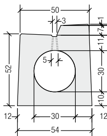
Profil P30RA7
