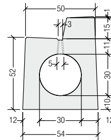
Profil P30RA15
