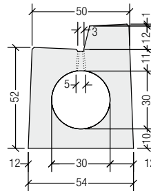
Profil P30RA12
