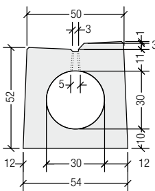
Profil P30RA3
