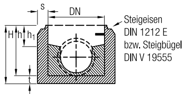
FT-Schacht DN 1000 bis Anschluss DN 600
